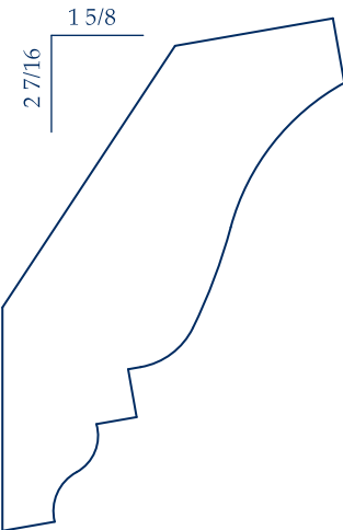
IL 313 13/16 x 2 7/8
