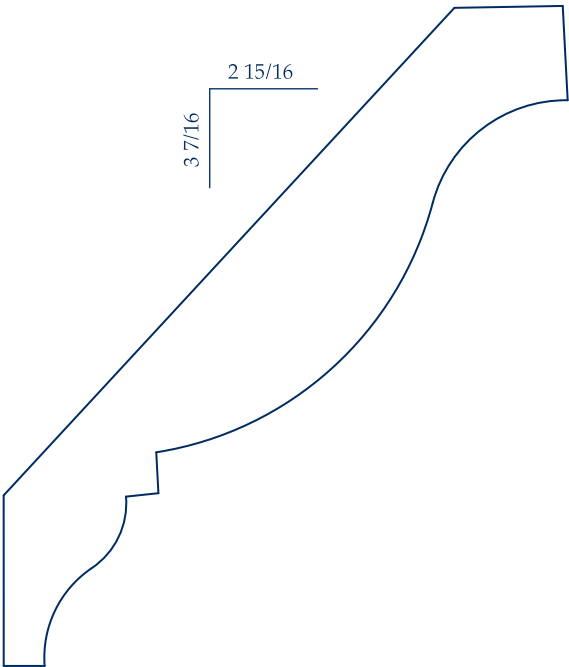
IL 386 13/16 x 4 1/2
