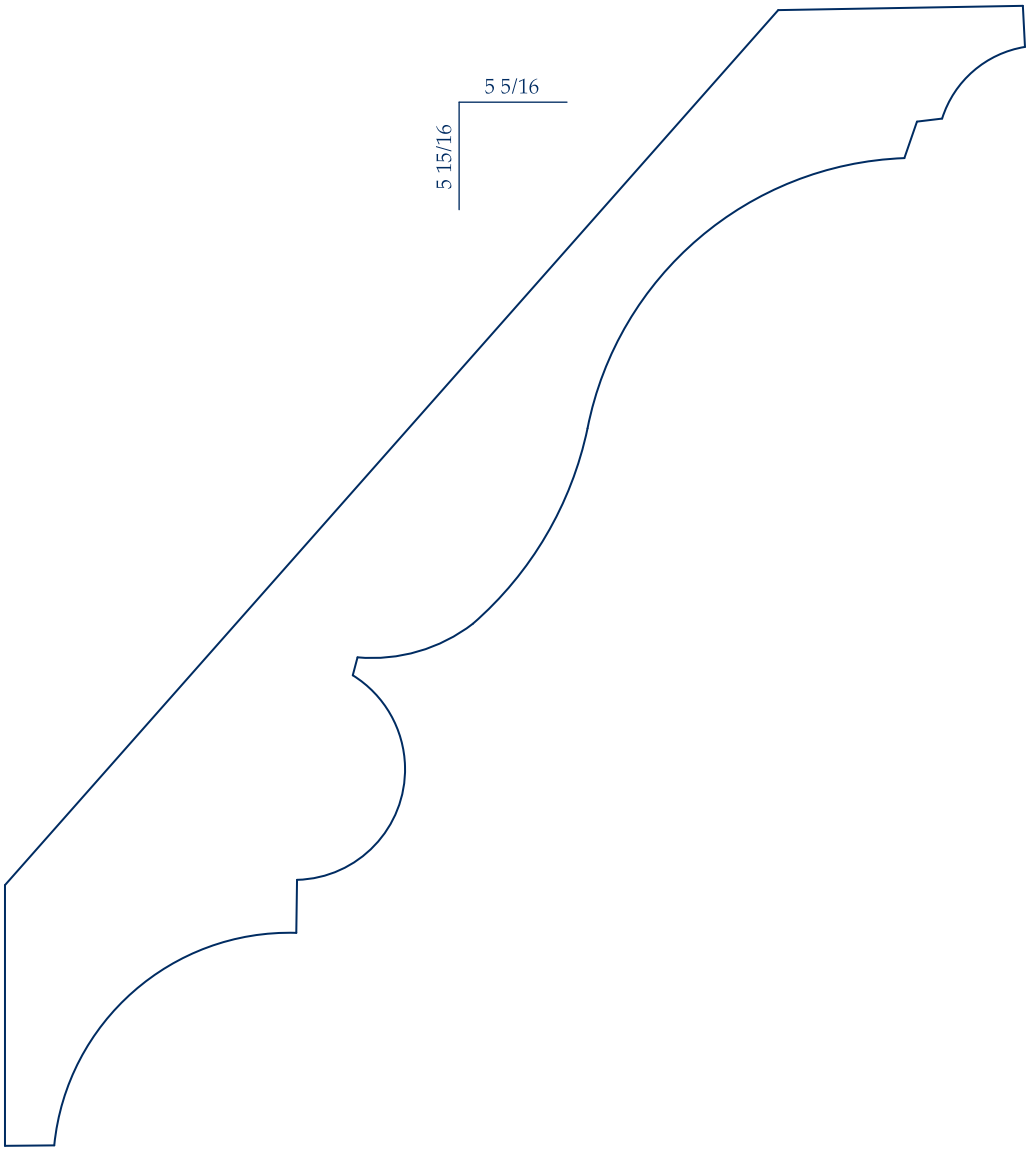
IL 392 1 5/16 x 8
